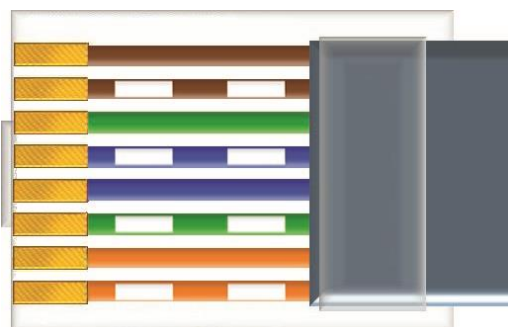
Обжим коннектора RJ-45 на 4-ех витых парах
