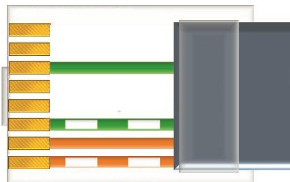
Обжим коннектора RJ-45 на 2-ух витых парах
